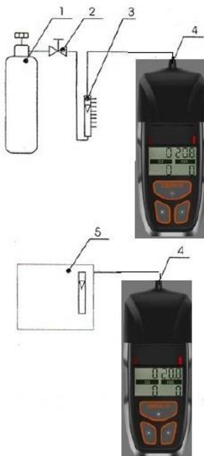
Рис. 1. - Схема соединения газоанализатора с источником ПГС
